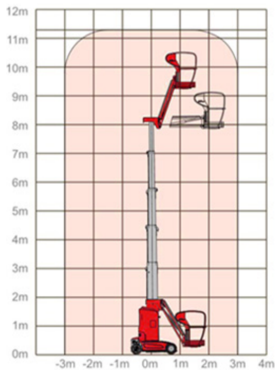
Arbeitsdiagramm Reichweite
